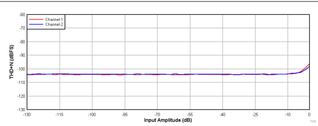
9-7. PCM1821-Q1: THD+N vs Input Amplitude
