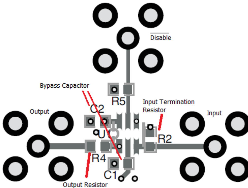
図 7-12. SBOS293 Layout
