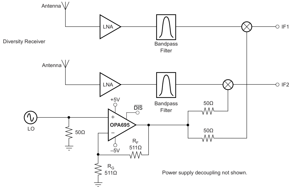
7-5. Dual Output LO Buffer
