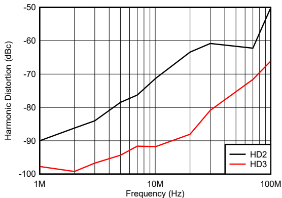
周波数に対する +8V/V ゲインでの高調波歪み
