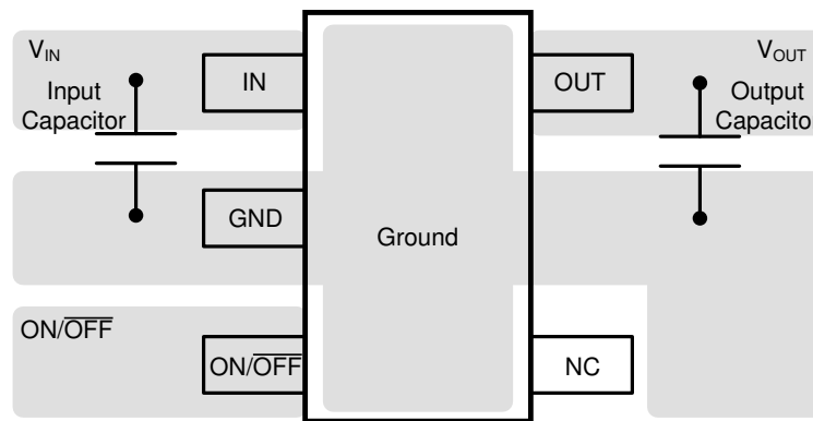
図 9-1. LP2981-N Layout Example
