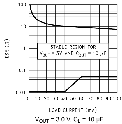
図 7-6. 3.0-V, 10- \mu F ESR Curves (Legacy Chip)
