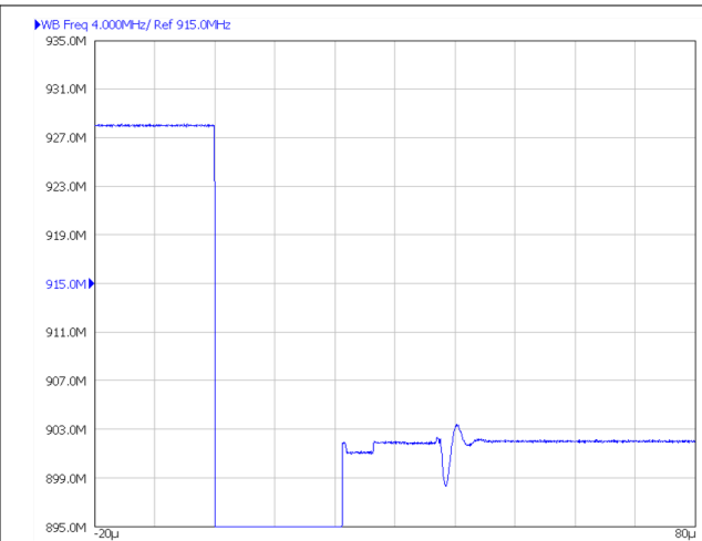
8-17. F2 (RX) to F1 (TX) Switching
