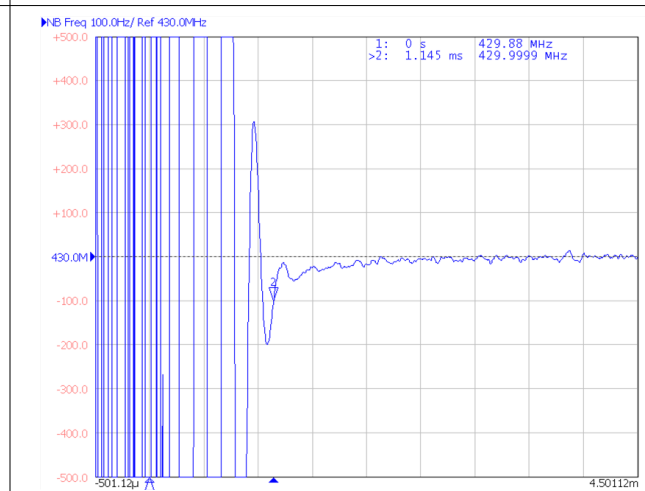
图 8-27. F2 to F1 Switching Time
