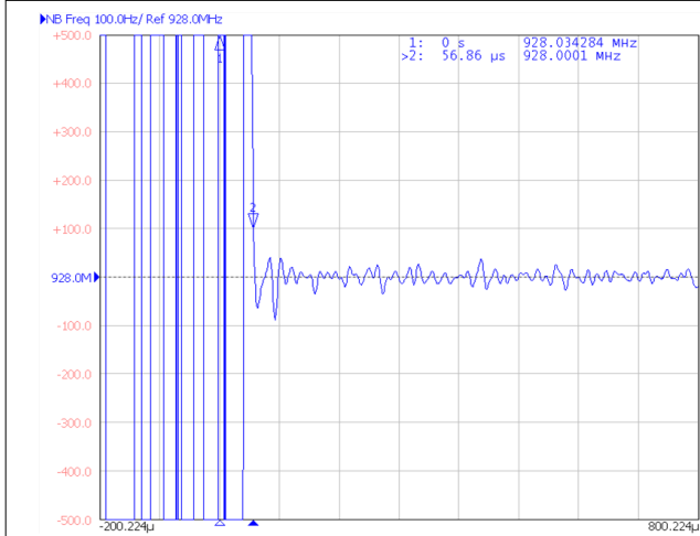
8-18. F1 to F2 Switching Time
