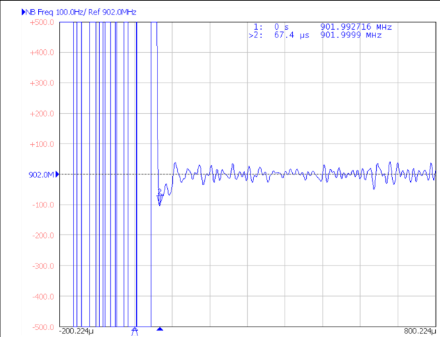
8-19. F2 to F1 Switching Time
