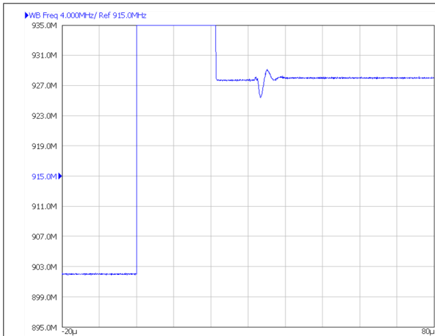
8-16. F1 (TX) to F2 (RX) Switching
