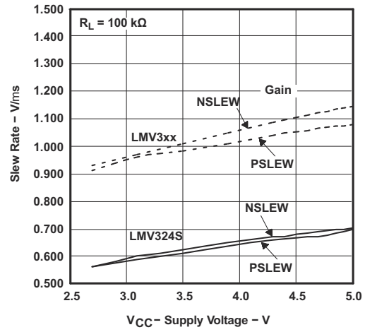
図 6-10. スルーレートと電源電圧との関係
