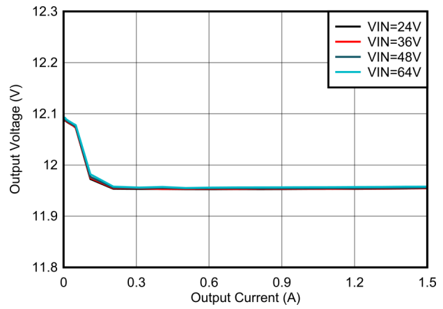
LMR38015-Q1 V_{OUT} = 12V 400kHz PFM バージョン
