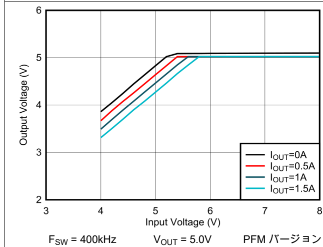
図 6-3. 5V ドロップアウト
