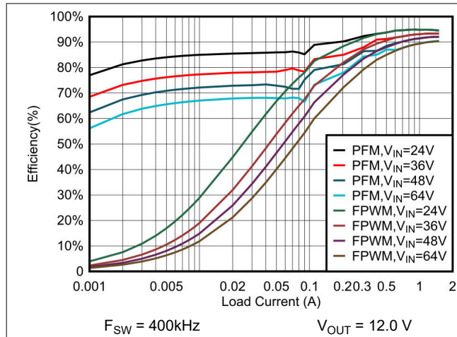
図 6-1. 効率と負荷電流との関係
