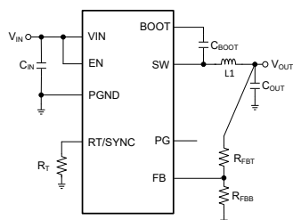
概略回路図
