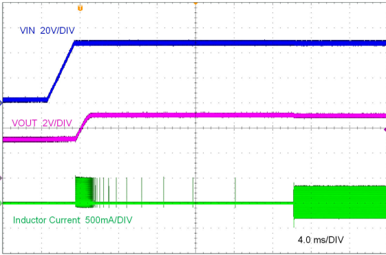
LMR38015-Q1 V_{OUT} = 5V 無負荷 3Vのバイアス
