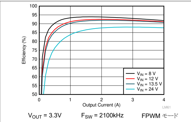
図 9-6. LMQ62440-Q1 の効率
