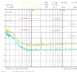
伝導 EMI : V_{\text{OUT}} = 5\text{V} 、 I_{\text{OUT}} = 4\text{A}
