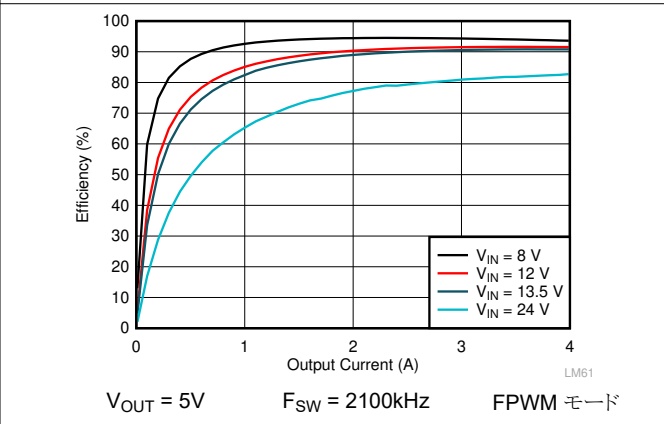
図 9-8. LMQ62440-Q1 の効率
