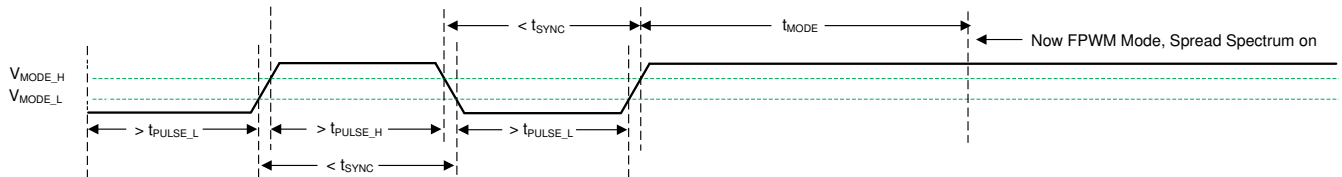
図 8-11. 同期モードから FPWM モードへの遷移
