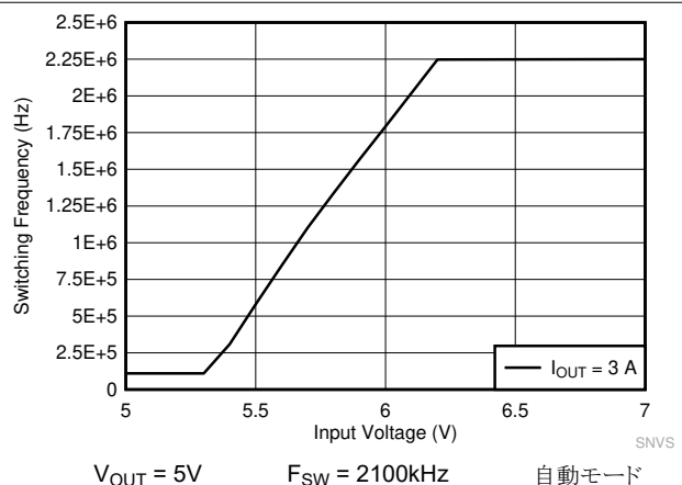
図 9-16. LMQ62440-Q1 の周波数ドロップアウト曲線
