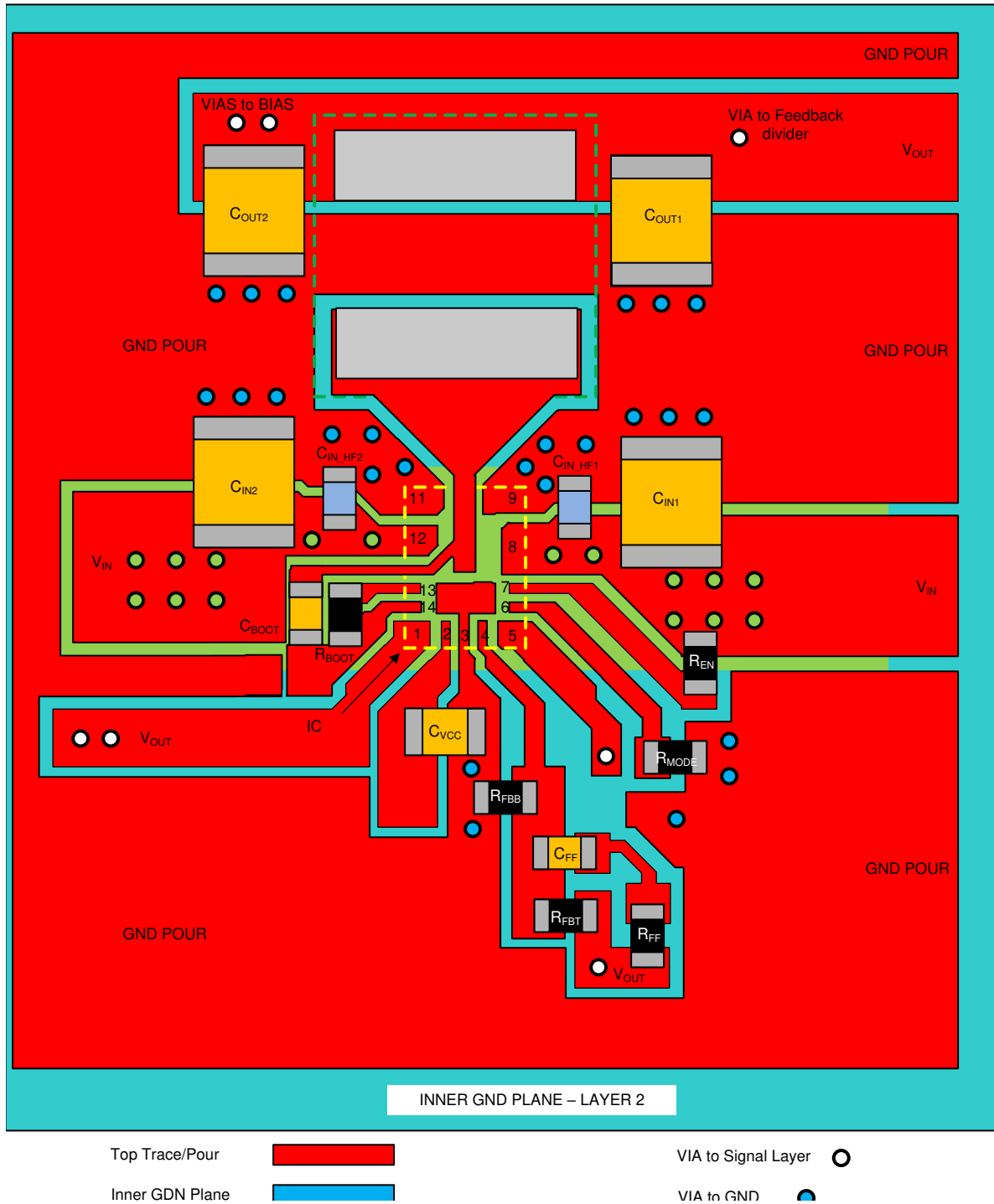
図 11-2. レイアウト例
