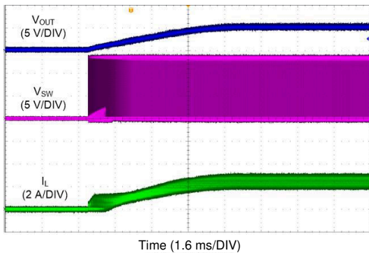
図 9-19. LMQ62440-Q1 の起動 (3.25A)
