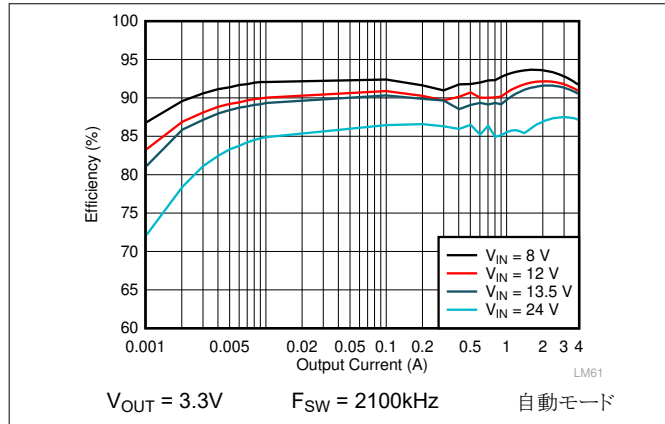
図 9-5. LMQ62440-Q1 の効率
