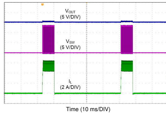
図 9-22. LMQ62440-Q1 の短絡特性
