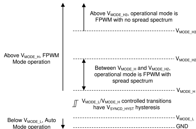
図 8-2. レベル依存モード選択設定
