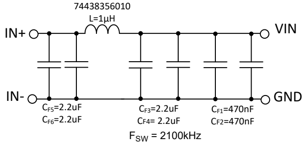
図 9-41. 推奨入力 EMI フィルタ
