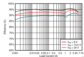
効率 : V_{\text{OUT}} = 5\text{V} 、 F_{\text{sw}} = 2.1\text{MHz}
