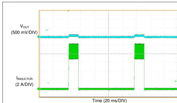
図 8-20. ヒックアップ中のインダクタ電流バースト
