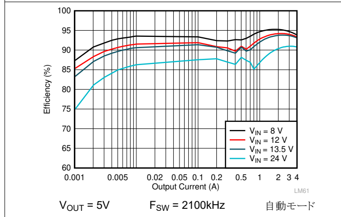
図 9-7. LMQ62440-Q1 の効率
