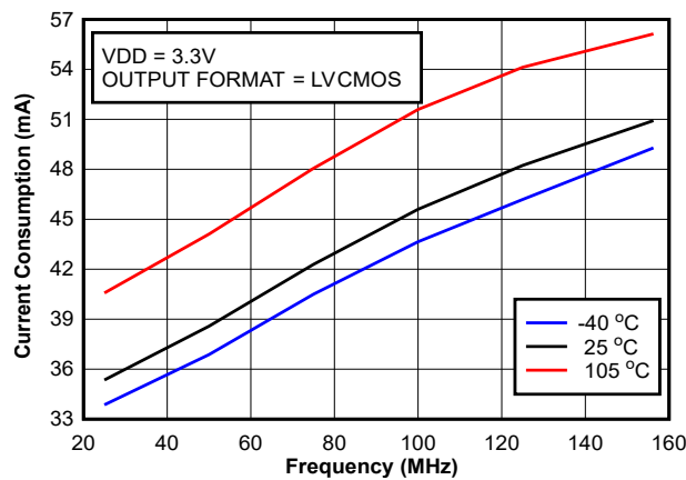
図 6-5. 消費電流と周波数との関係 (LVC MOS、3.3V)
