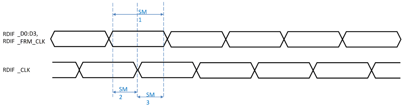
図 7-17. RDIF のタイミング要件
