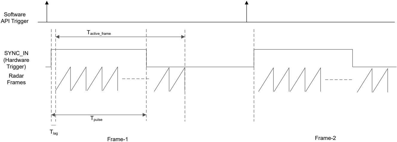
図 7-11. 同期入力ハードウェア トリガ
