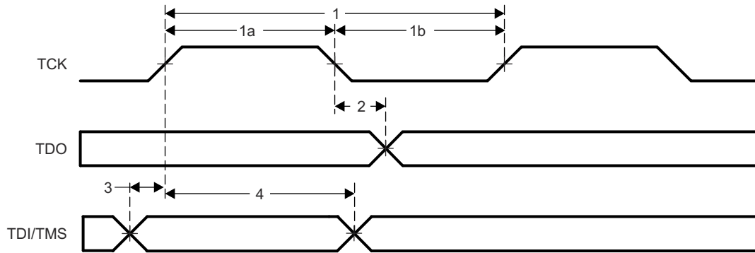
図 7-22. JTAG のタイミング
