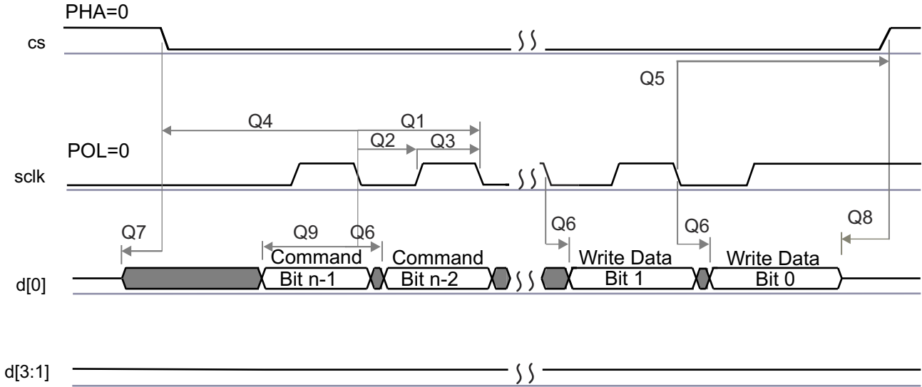
図 7-21. QSPI 書き込み (クロック モード 0)
