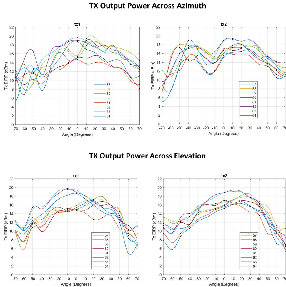
図 7-8. トランスミッタのアンテナ放射パターン
