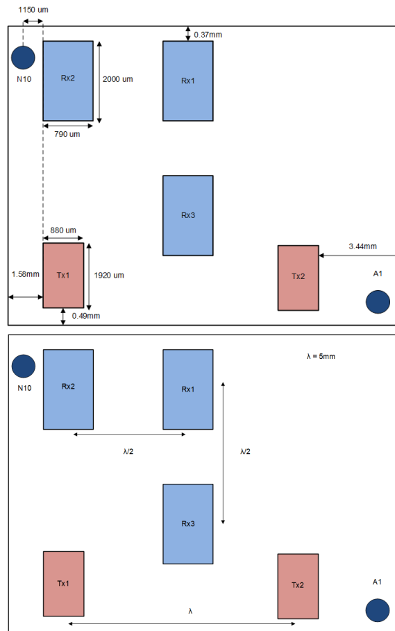
図 7-9. アンテナ位置 (配置と相対間隔)
