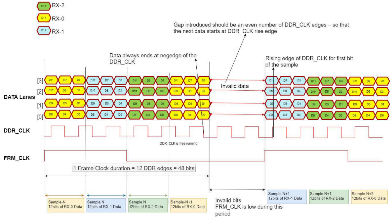
図 7-18. RDIF データ形式
