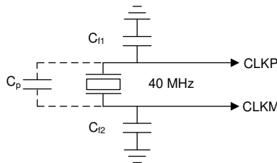
図 7-12. 水晶振動子の実装
