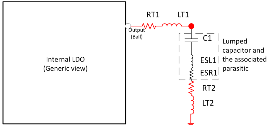
図 7-4. 出力パスの各部分が持つ寄生素子 (コンデンサが 1 つの場合)
