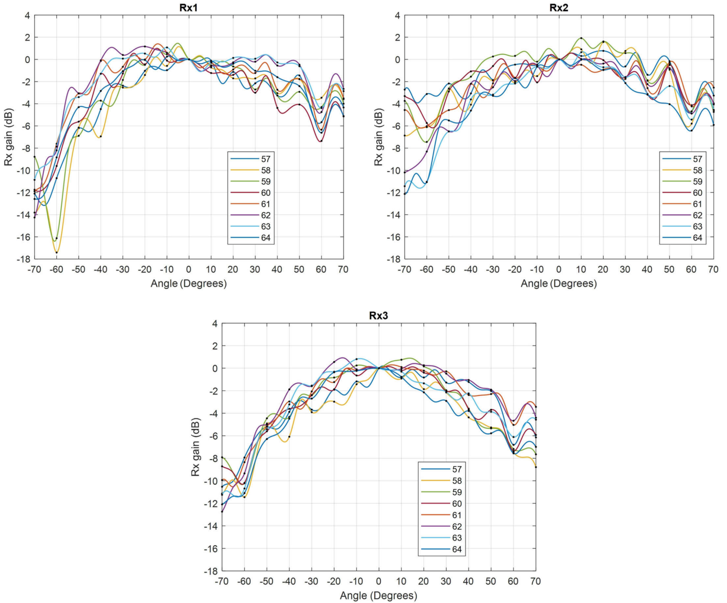
図 7-7. ボアサイト ゲインで正規化されたレシーバ アンテナ視野角 (FOV)
