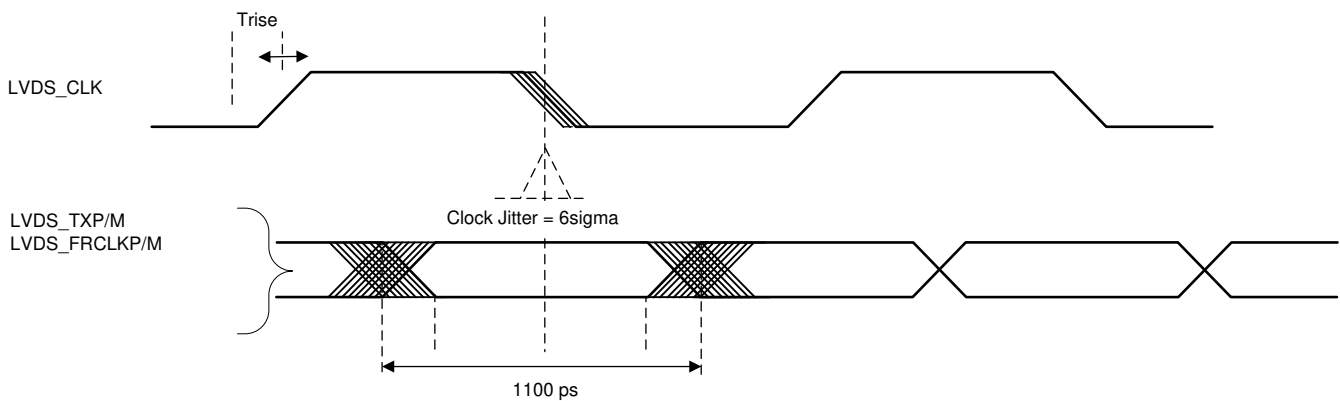
8-11. Timing Parameters
