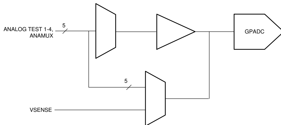
9-6. ADC Path
