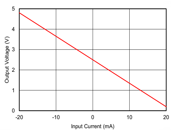
図 9-5. PLC の出力電圧と入力電圧との関係
