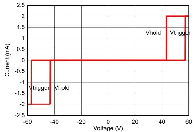
图 5-2. DC I-V Curve
