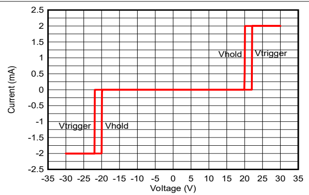
図 5-2. DC I-V Curve
