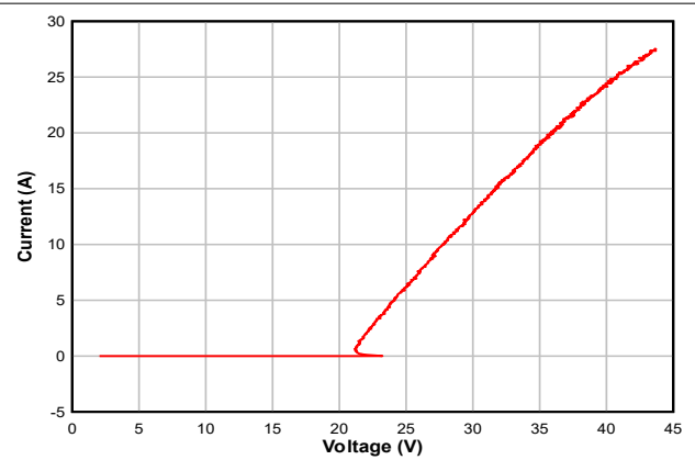
図 5-4. Negative TLP Curve
