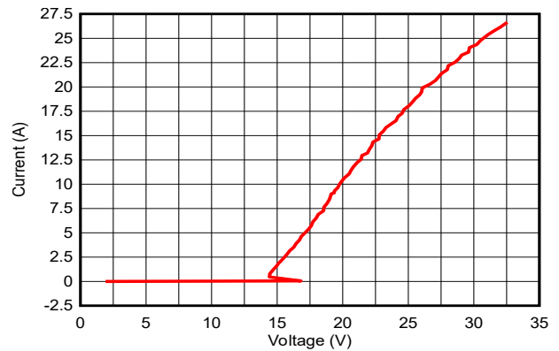
図 5-4. Negative TLP Curve
