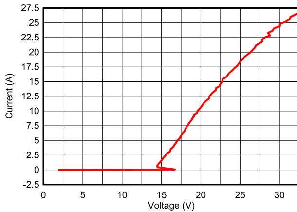
図 5-3. Positive TLP Curve
