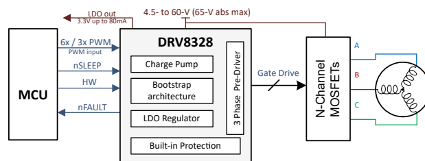
DRV8328 の概略回路図
