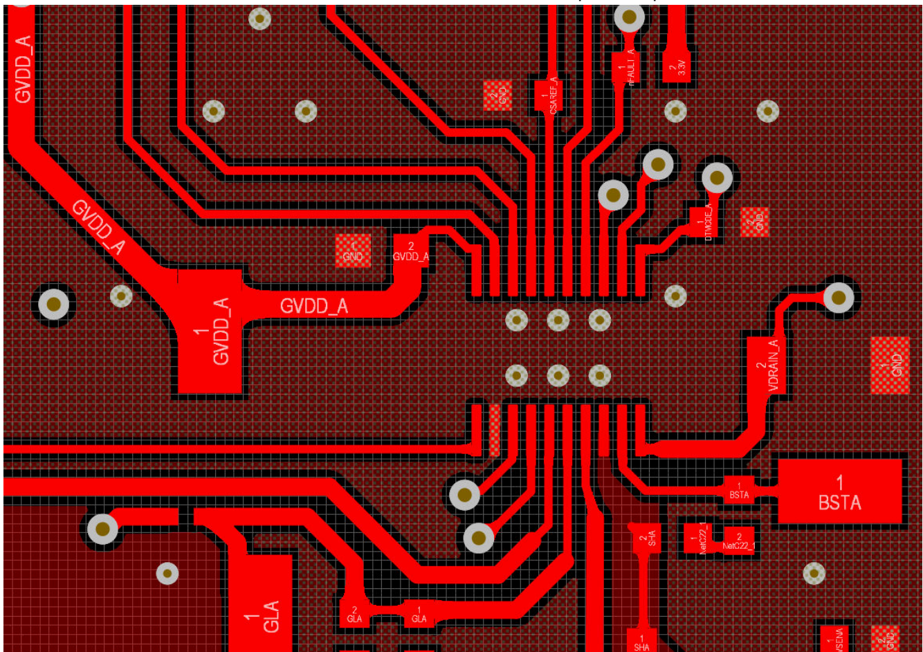
図 9-1. DRV8161 Layout
