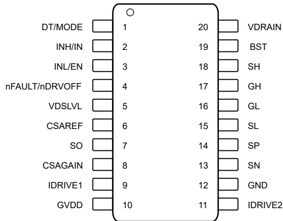
図 5-1. DRV8161 DGS Package 20-pin VSSOP Top View
