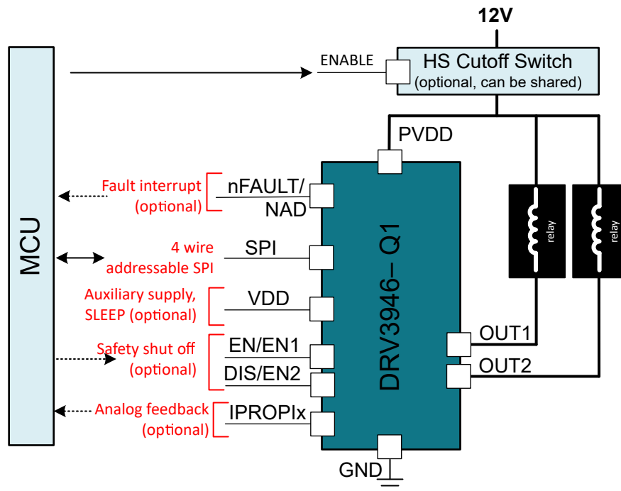
概略回路図
