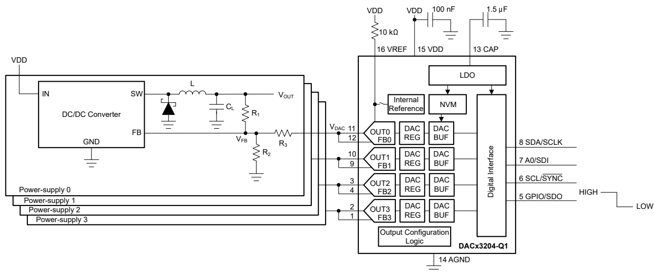
図 8-1. APD Biasing
