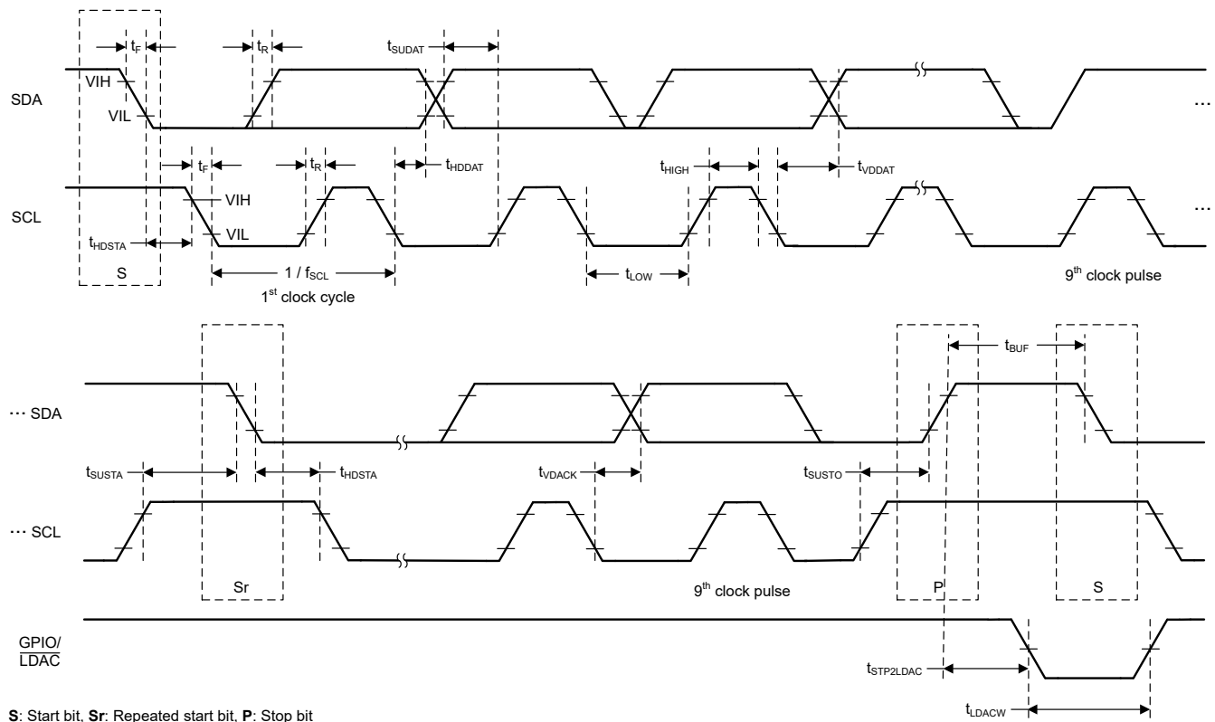
图 5-1. I 2 C Timing Diagram
