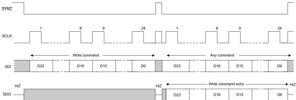
図 6-14. SPI Write Cycle
