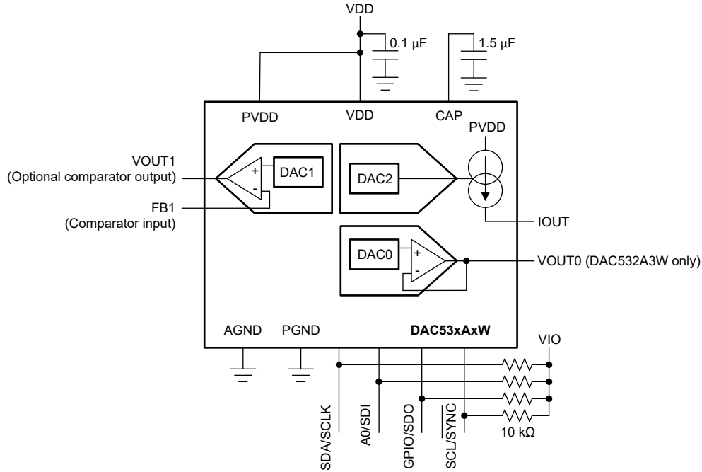
図 6-2. Comparator Interface
