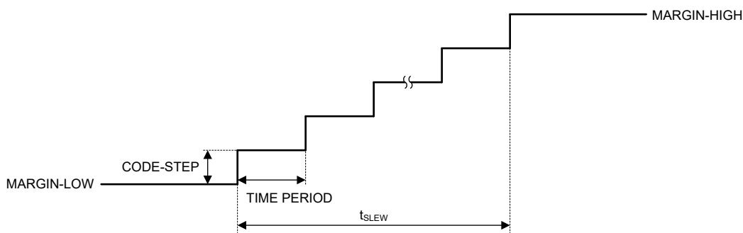
图 6-9. Programmable Slew-Rate Control
