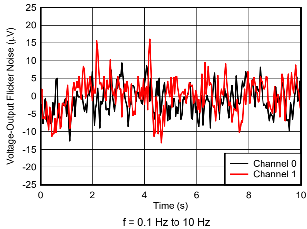
図 5-28. Voltage Output Flicker Noise
