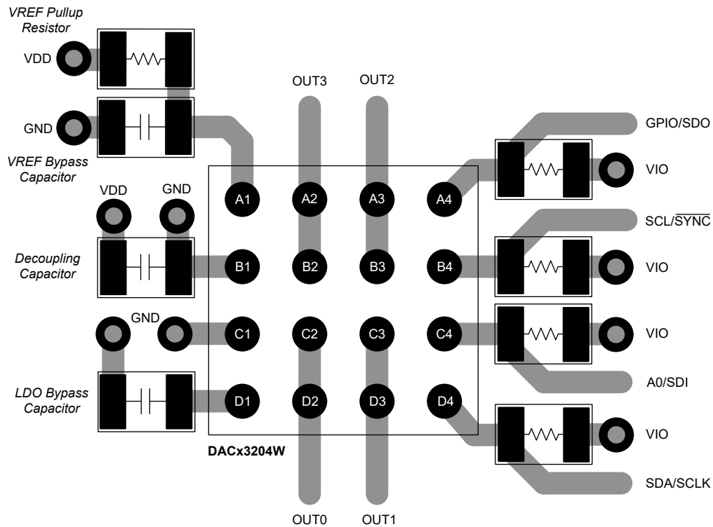
8-3. Layout Example
