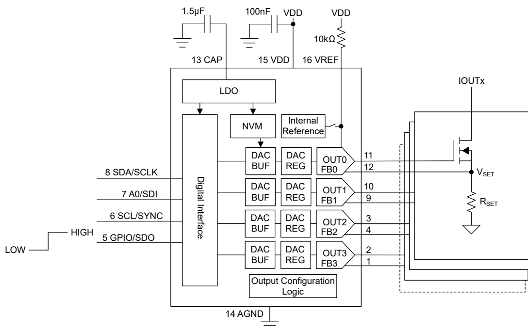
図 8-1. Current Source
