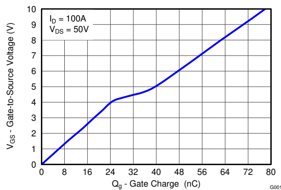
ゲート電荷
