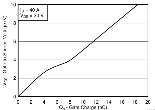
ゲート電荷
