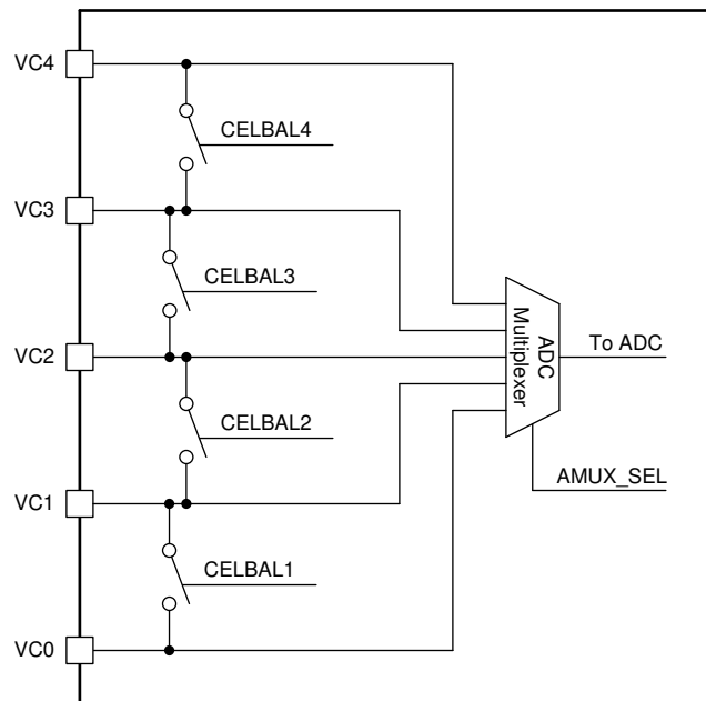
図 5-2. VCx Pins
