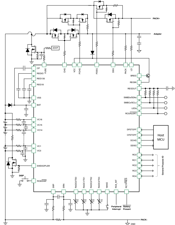
概略回路図
