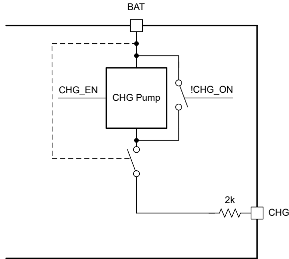
図 5-5. CHG Pin
