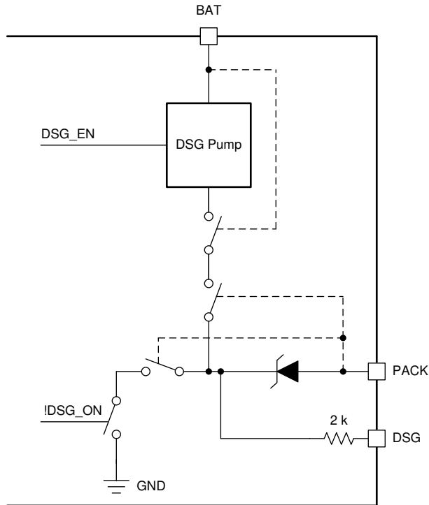
図 5-6. DSG Pin
