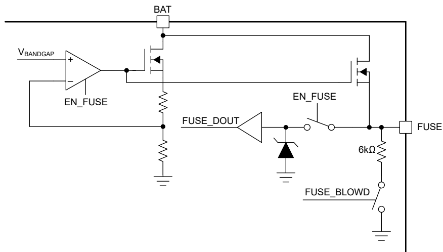
図 5-4. Fuse Pin
