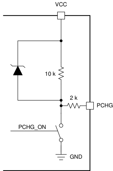
5-7. PCHG Pin
