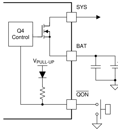
图 9-11. QON 电路
