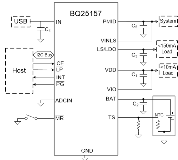
概略回路図
