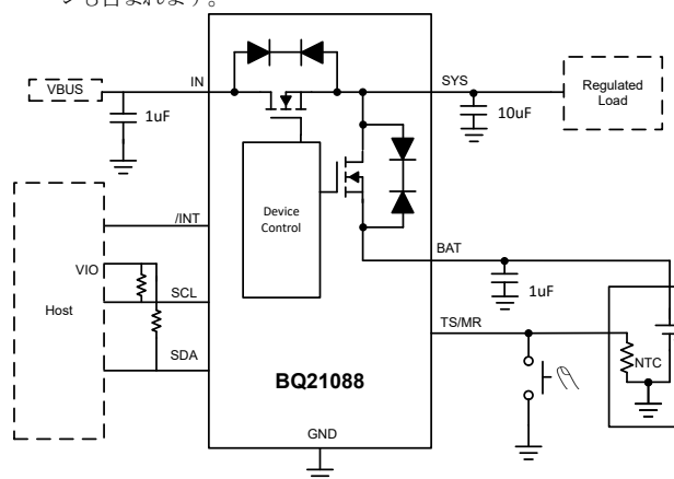
概略回路図
