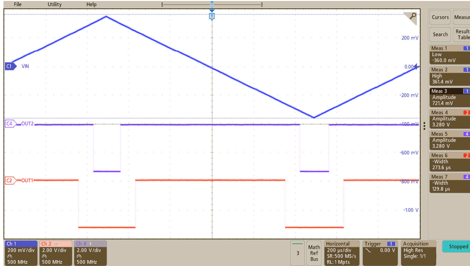
図 7-2. 三角入力波に対する AMC23C15 -Q1 の出力応答
