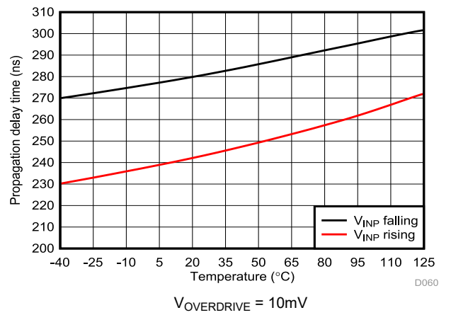
図 5-51. Cmp3 の伝搬遅延と温度との関係
