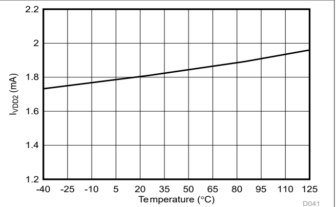
図 5-61. ハイサイド電源電流と温度との関係
