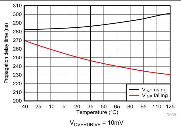
図 5-49. Cmp2 の伝搬遅延と温度との関係
