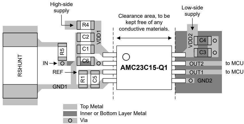
図 7-8. AMC23C15 -Q1 の推奨レイアウト
