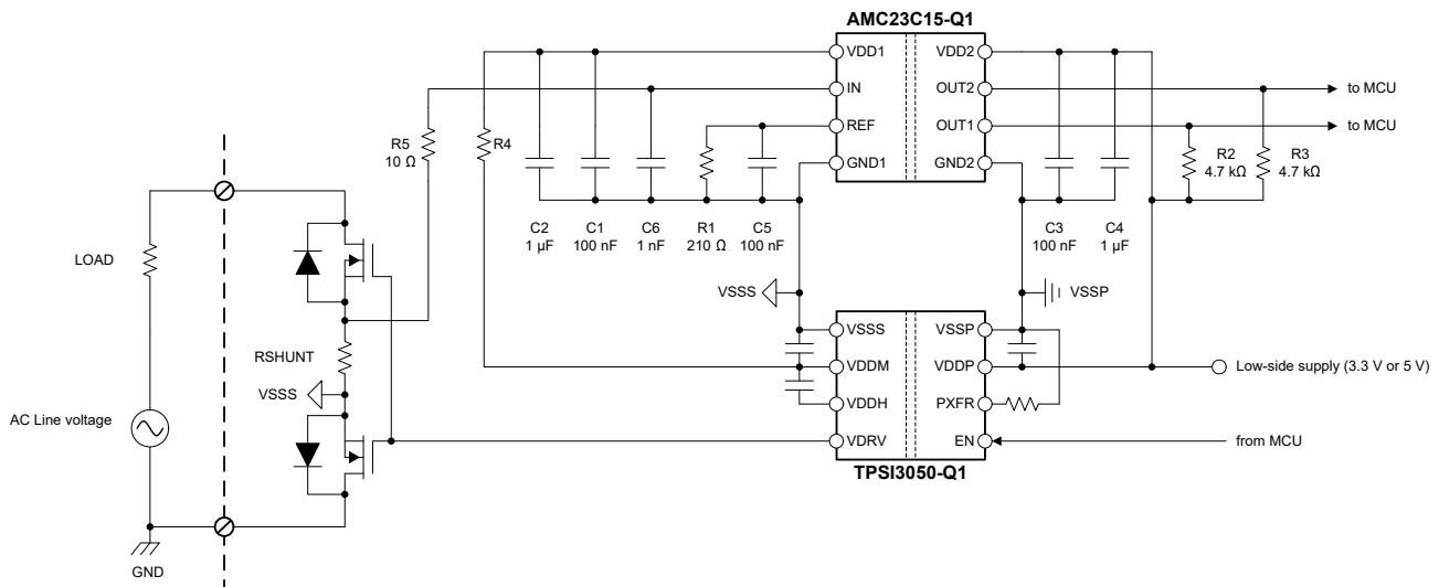
図 7-1. AMC23C15-Q1 による過電流および短絡の検出
