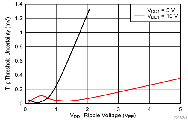
図 7-6. VDD1 リップル電圧に対するトリップ スレッシュホルド感度 (Cmp3、 f_{\text{RIPPLE}} = 10\text{kHz} )
