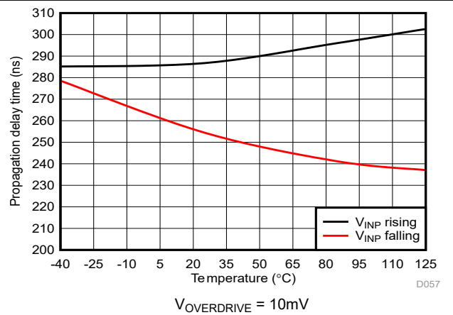
図 5-53. Cmp0 の伝搬遅延と温度との関係
