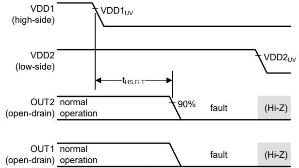
図 6-8. VDD1 がオフになってから VDD2 がオフになる
