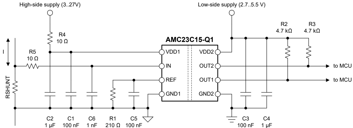
図 7-7. AMC23C15-Q1 のデカップリング
