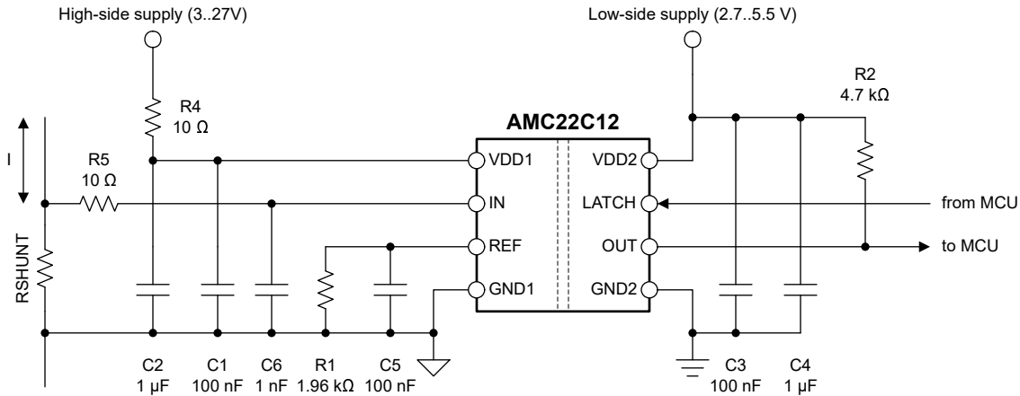
図 7-6. AMC22C12 のデカップリング
