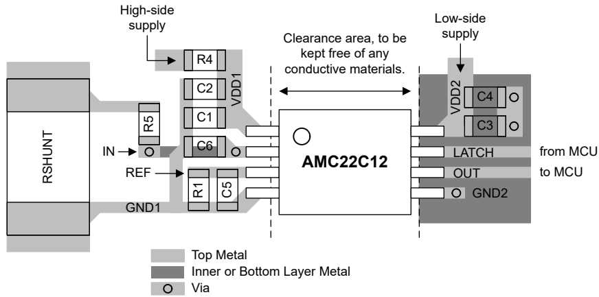
図 7-7. AMC22C12 の推奨レイアウト
