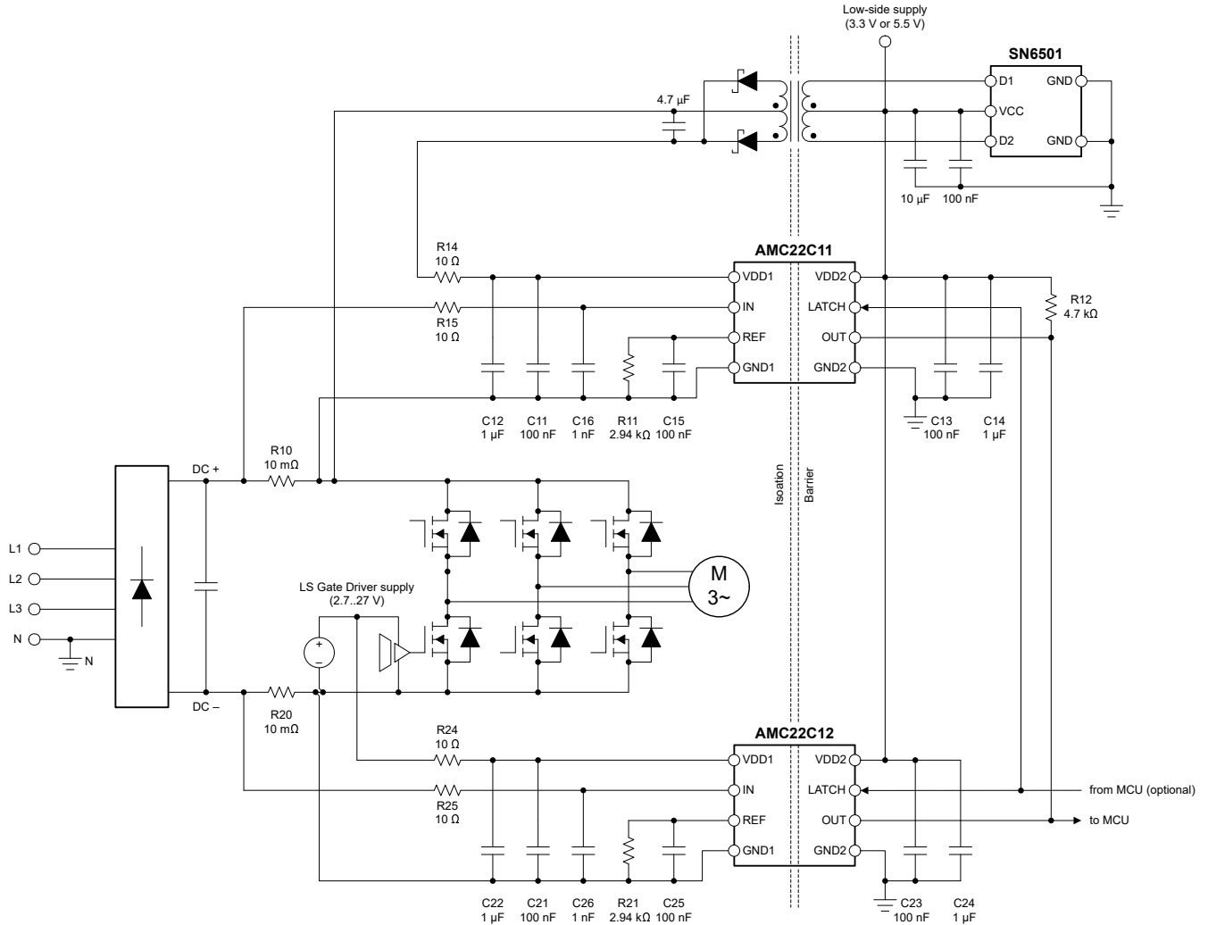
図 7-1. AMC22C11 による DC+ 過電流検出
