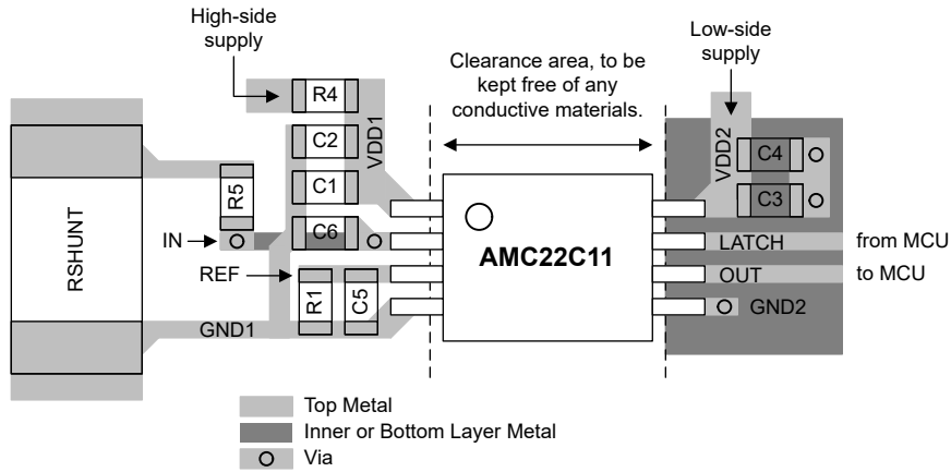
図 7-5. AMC22C11 の推奨レイアウト
