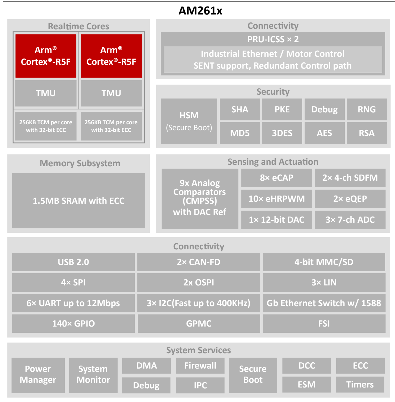
図 3-1. AM261x の機能ブロック図
