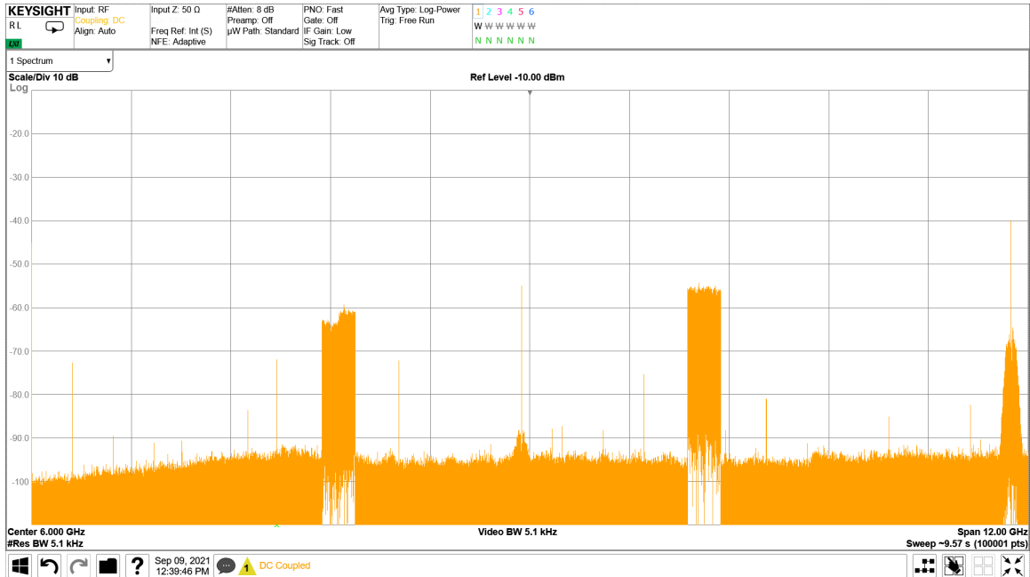
4-232. TX 4x100MHz NR Output Spectrum 8.11GHz
