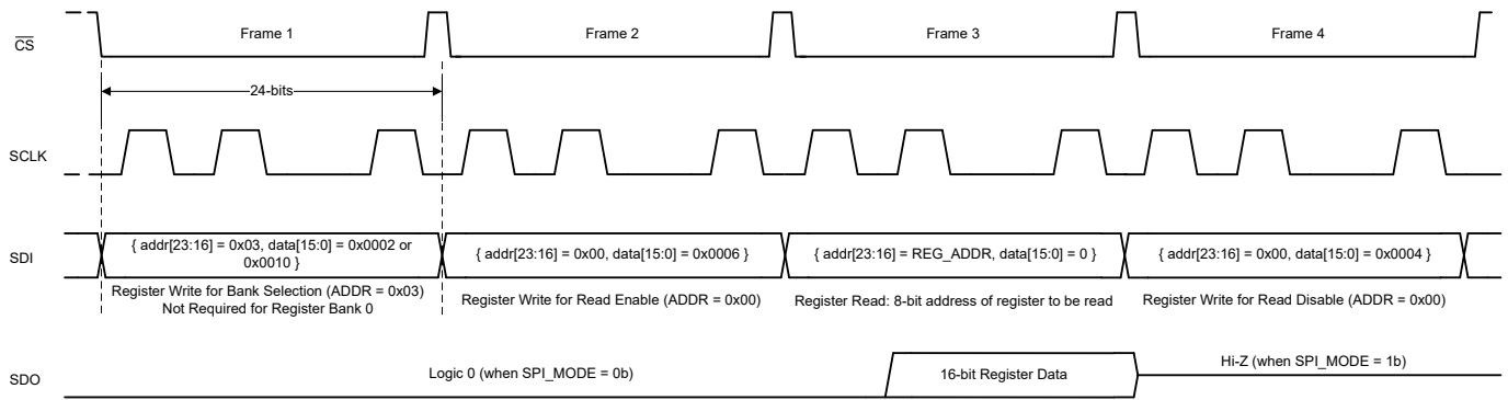
图 6-10. Register Read
