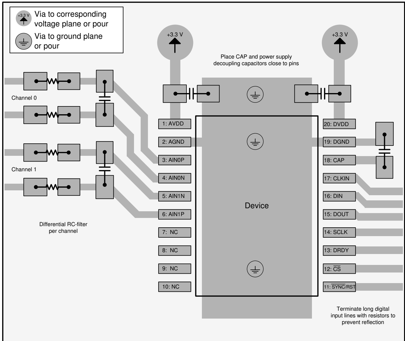
9-6. Layout Example
