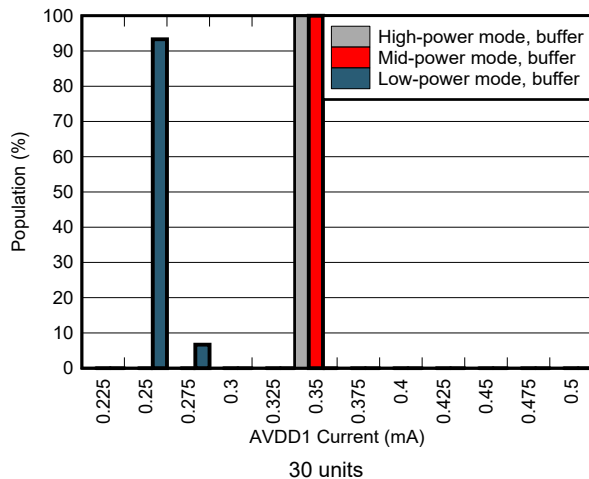
6-61. AVDD1 Current Distribution
