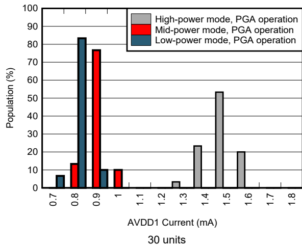
6-60. AVDD1 Current Distribution
