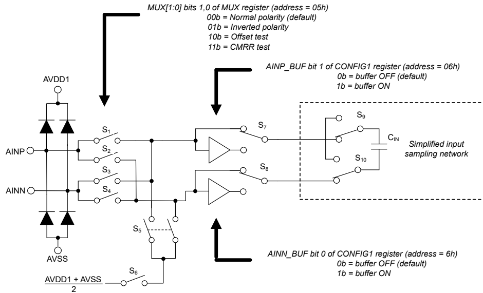
图 7-3. Analog Input Circuit
