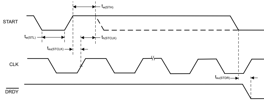
图 5-6. START Pin Timing
