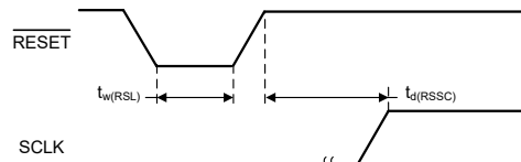
图 5-5. RESET Pin Timing
