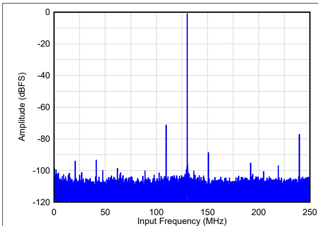
図 9-4. FFT1 : DDC バイパス、 A_{\text{IN}} = -1\text{dBFS}
