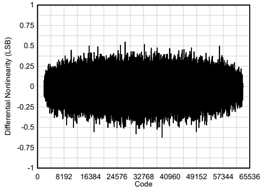
図 6-23. DNL
