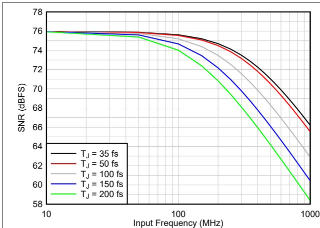
図 9-2. SNR と T_{\text{Jitter}} と F_{\text{IN}} との関係
