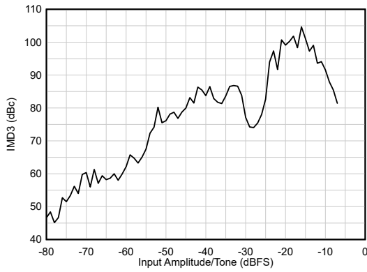
図 6-17. IMD3 と A_{IN} との関係 F_{IN} = 70/100\text{MHz}
