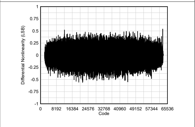
図 6-50. DNL
