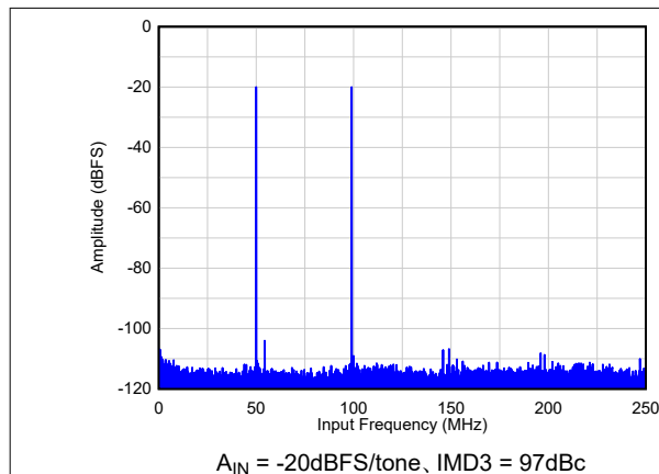
図 6-39. F_{IN} = 401/450\text{MHz} での 2 トーン FFT
