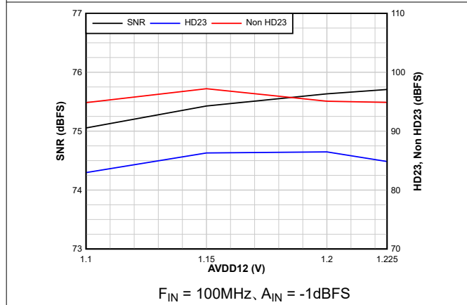
図 6-47. AC 性能と AVDD12 との関係
