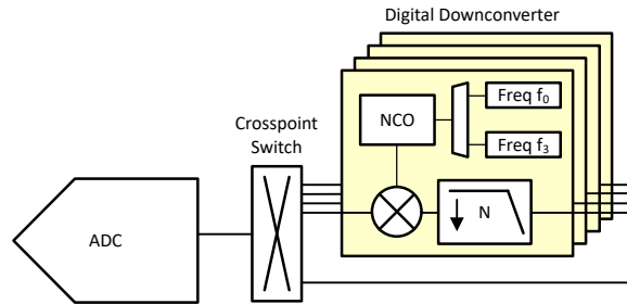
図 8-21. 内蔵デジタル ダウン コンバータ
