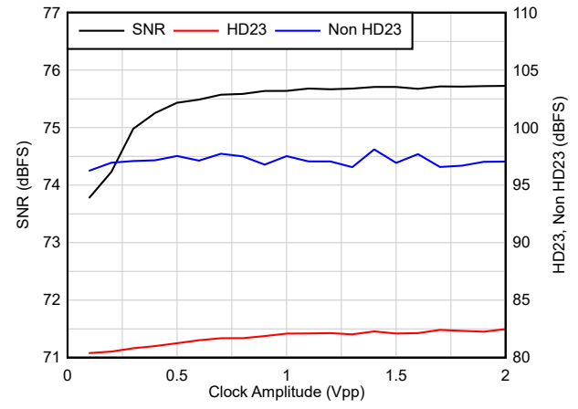
図 9-3. SNR とクロック振幅との関係 ( F_{\text{S}} = 500\text{MSPS} 、 F_{\text{IN}} = 100\text{MHz} 、 A_{\text{IN}} = -1\text{dBFS} )
