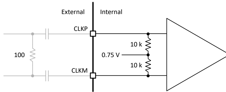
図 8-8. サンプリングクロック入力回路
