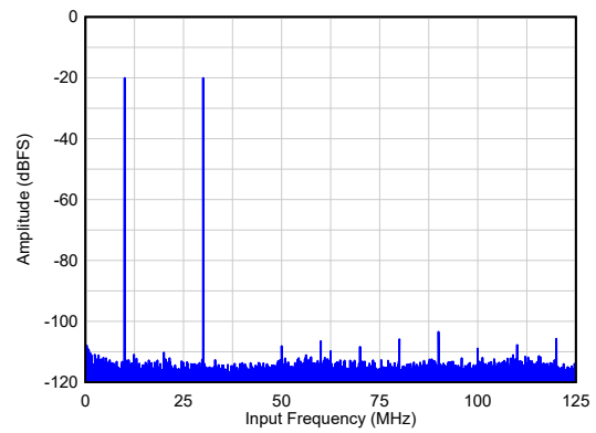
図 6-12. F_{IN} = 220/240\text{MHz} での 2 トーン FFT
