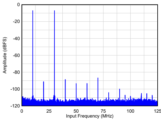
図 6-11. F_{IN} = 220/240\text{MHz} での 2 トーン FFT
