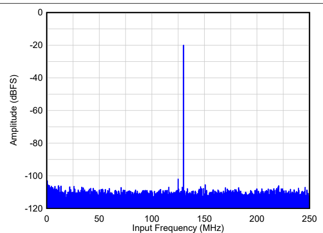
図 9-5. FFT2 : DDC バイパス、 A_{\text{IN}} = -20\text{dBFS}
