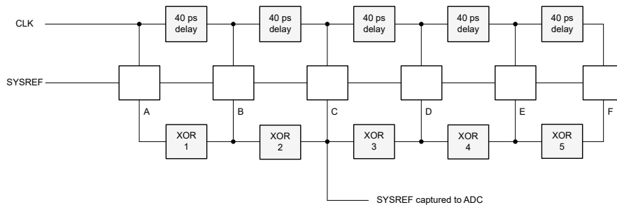
図 8-17. SYSREF 検出回路
