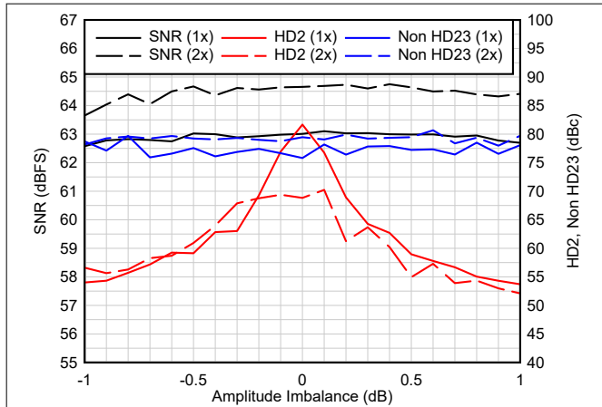
図 6-3. Amplitude Imbalance - 2.6 GSPS
