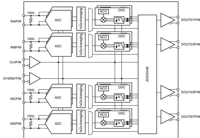
ブロック図
