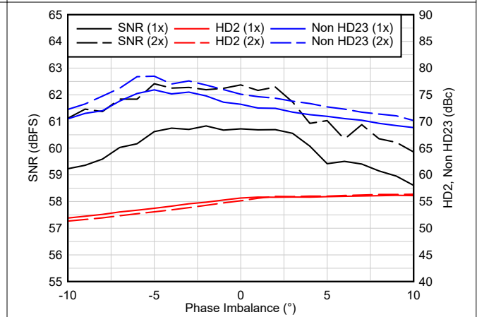
図 6-6. Phase Imbalance - 3.0 GSPS
