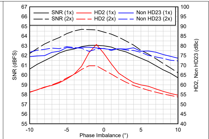
図 6-4. Phase Imbalance - 2.6 GSPS
