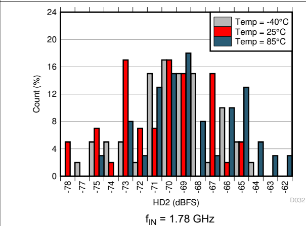
6-56. HD2 Histogram at AVDD19 = 1.9 V
