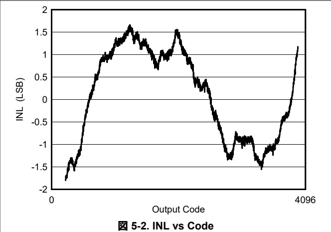
図 5-2. INL vs Code
